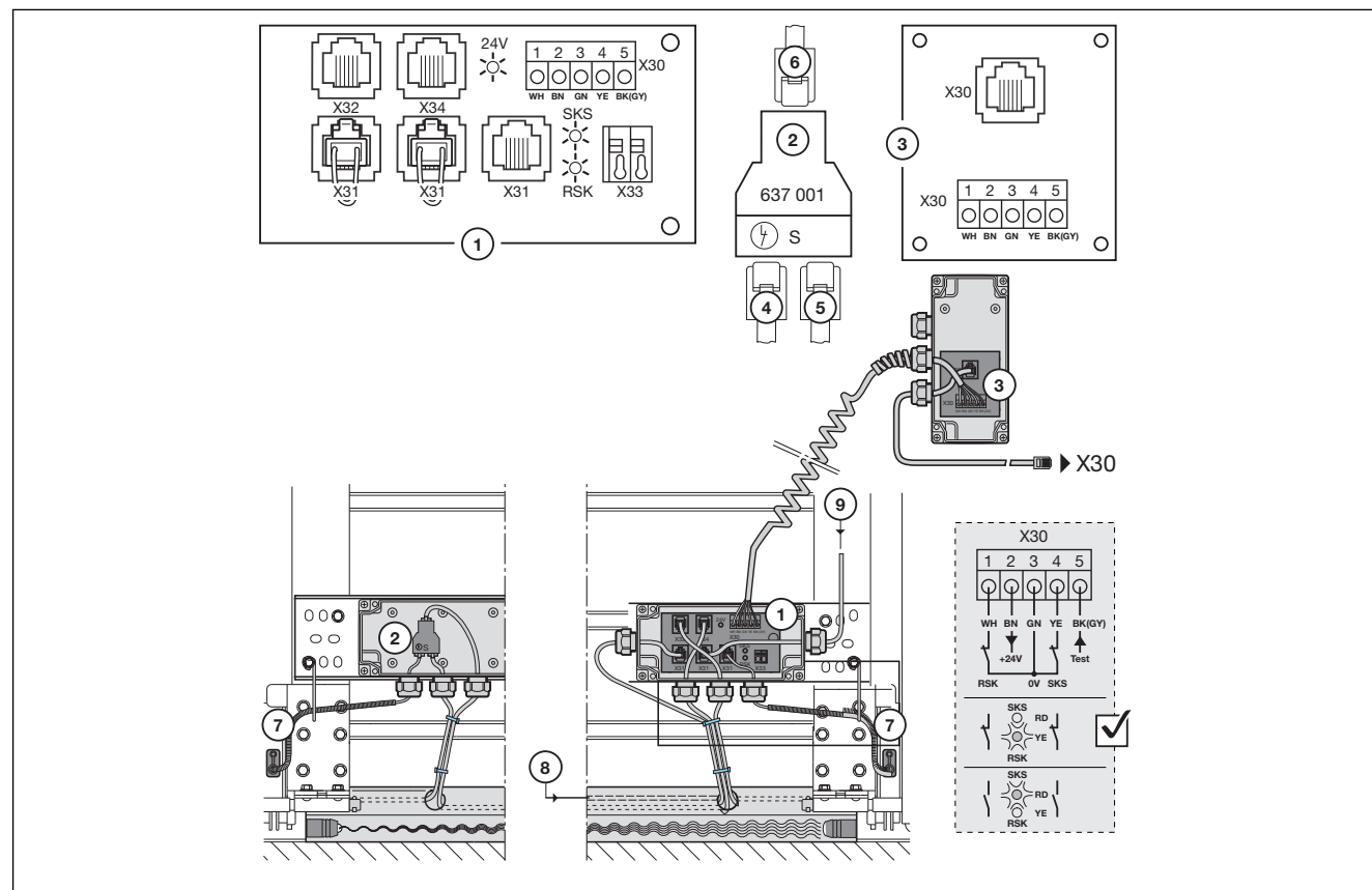
Abb. 7-4: Schließkantensicherung
