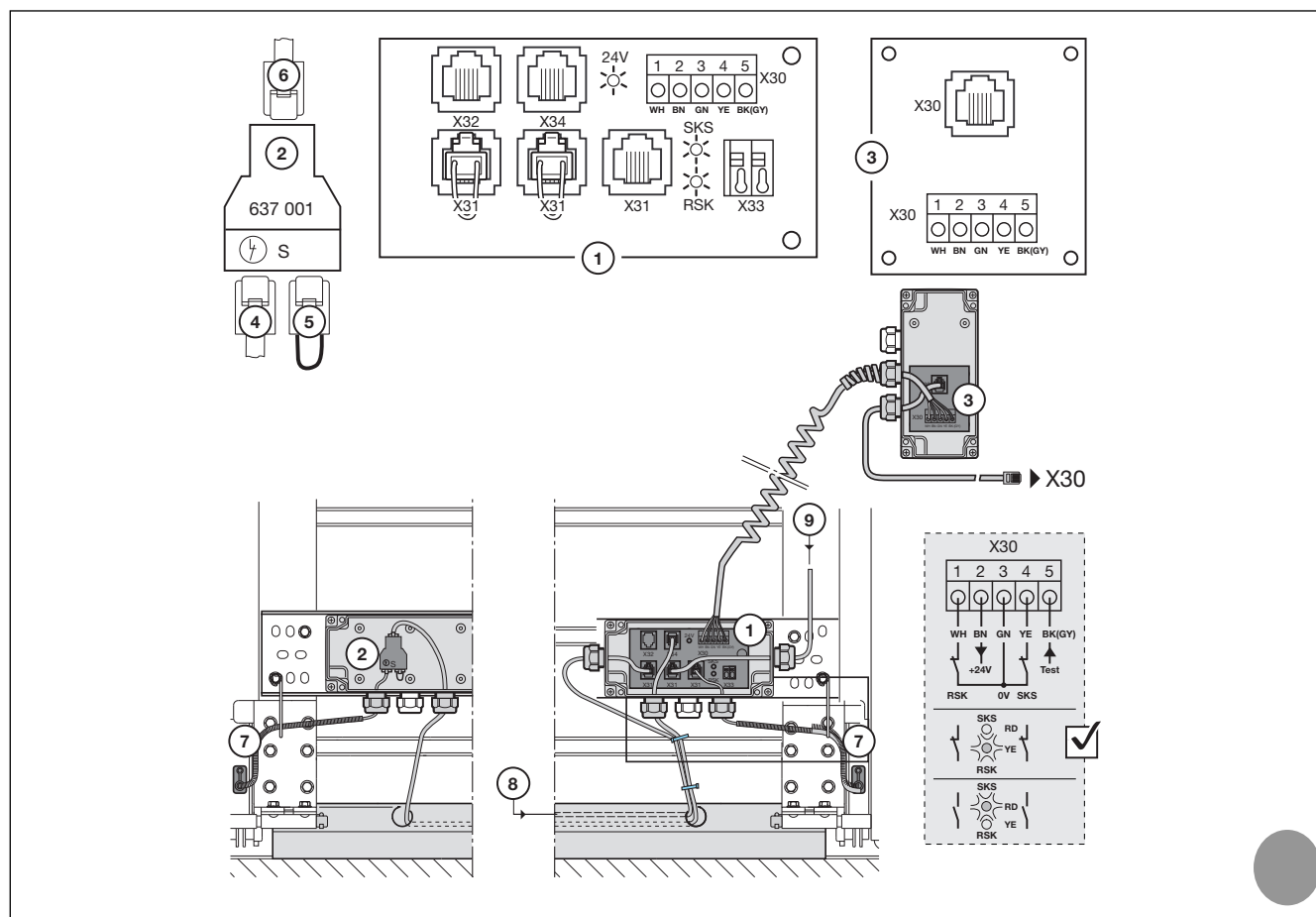
Abb. 7-6: Anschlusseinheit Totmann
