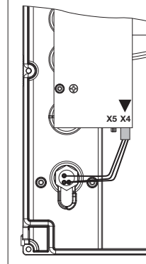
Abb. 6–28: Anschluss des Miniaturschlosses, Deckelinnenseite, von X5 nach X4 umstecken
