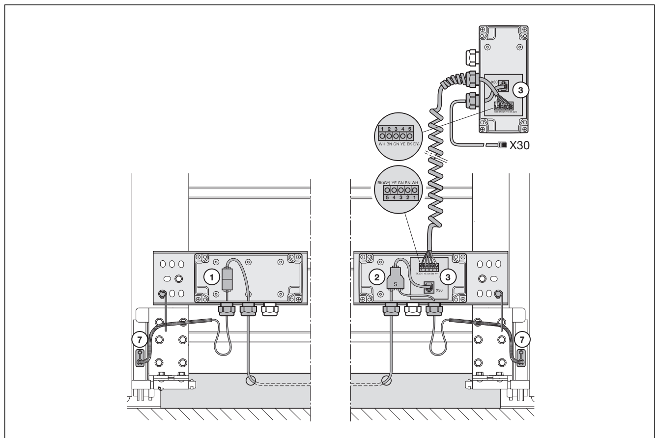
Abb. 7-5: Anschlusseinheit Totmann
