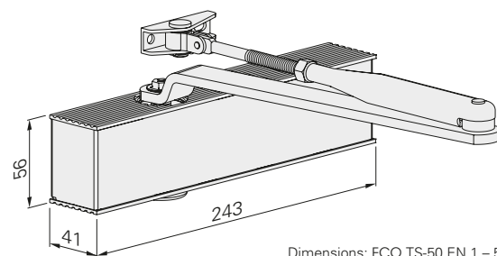
Dimensions: ECO TS-50 EN 1 – 5
