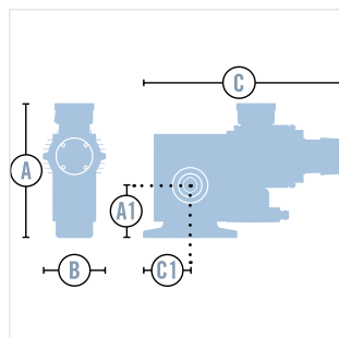
MTZ-FU 30 HD
